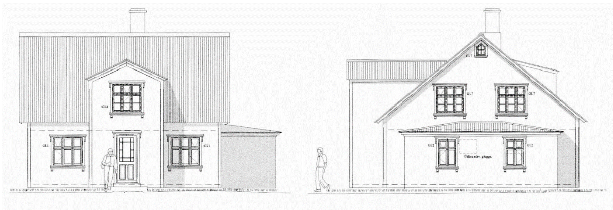
Mynd 2:2 Hlíðarhús, hluti útlitsteikninga. Höfundur Teiknistofan Skólavörðustíg 28.
